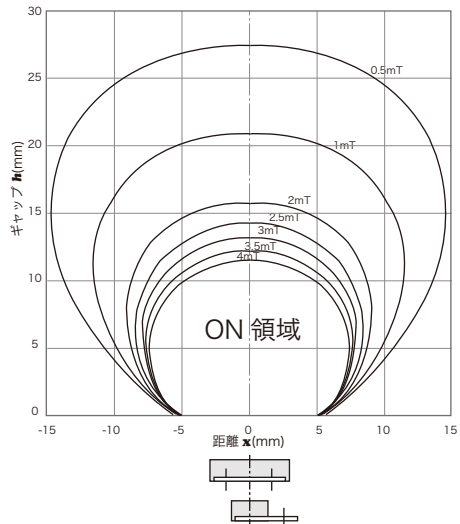
磁気特性
