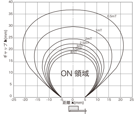
磁気特性
